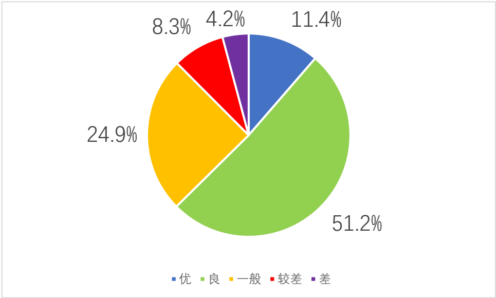
图 2 2022 年第三季度水环境指数不同等级城市数量占比
