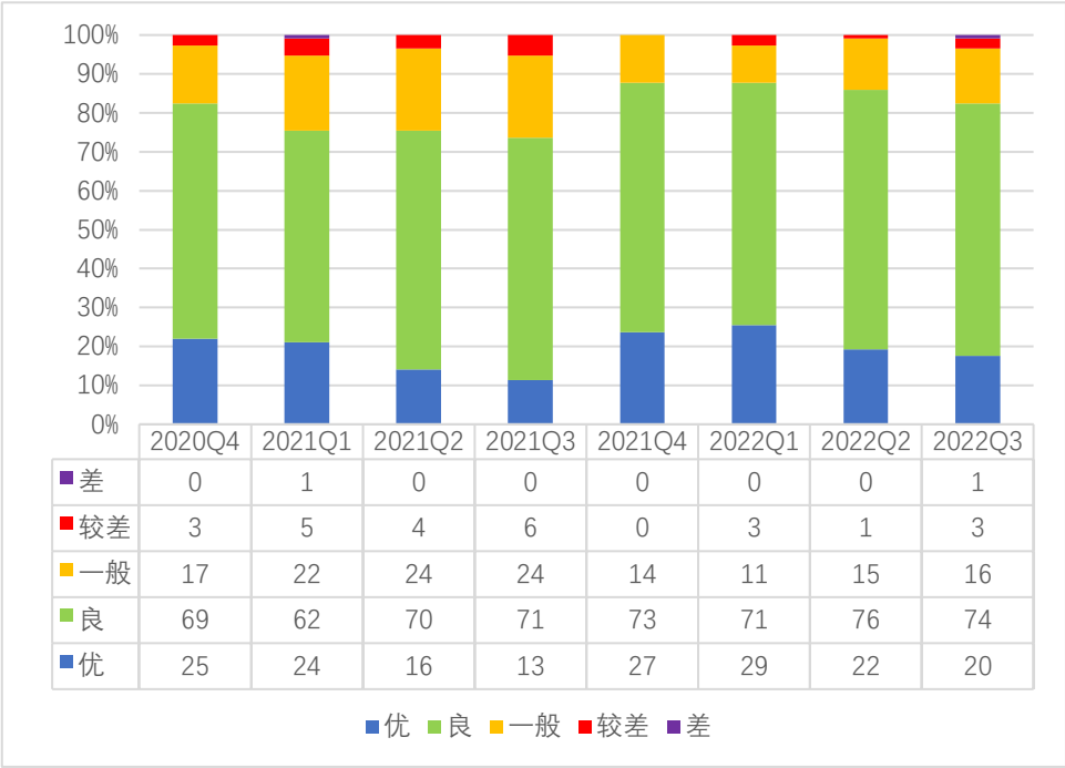
图 5 长江流域水环境指数不同等级城市数量同比和环比
