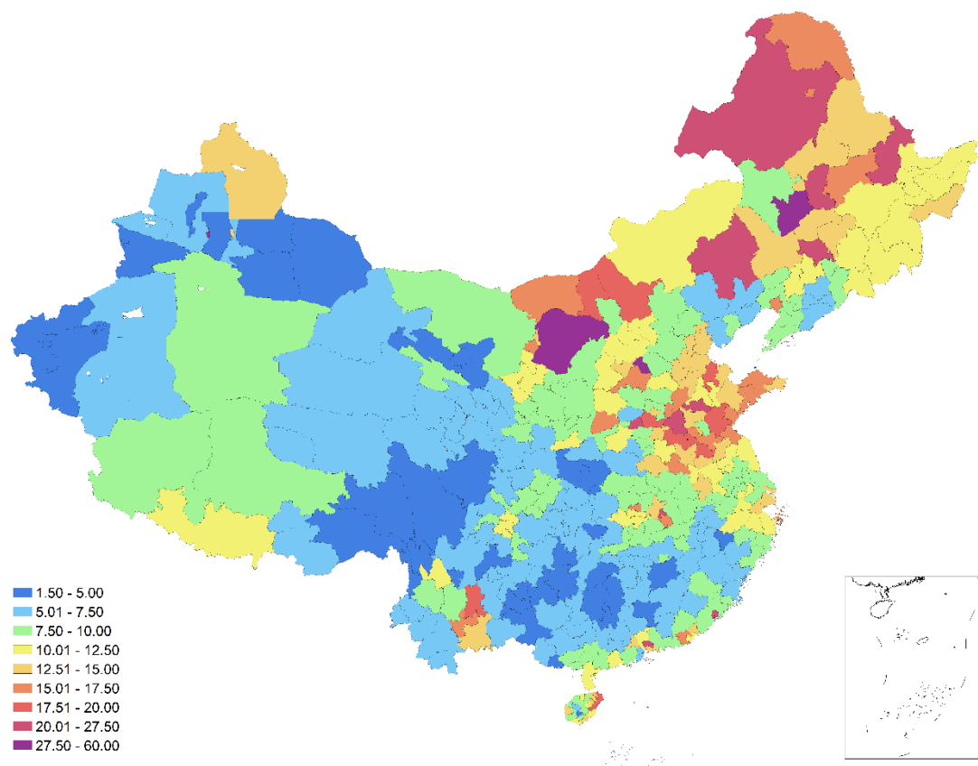
图 1 2022 年第三季度全国城市地表水水环境指数
